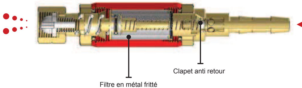
Filtre en métal fritté
