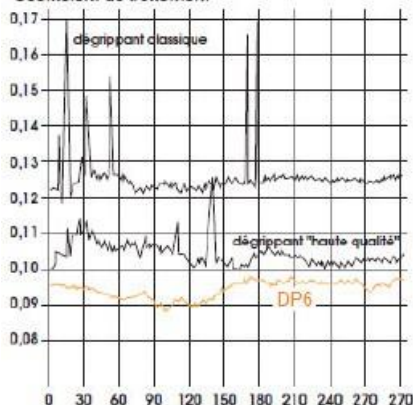
SRV : TEST DE FRICTION
